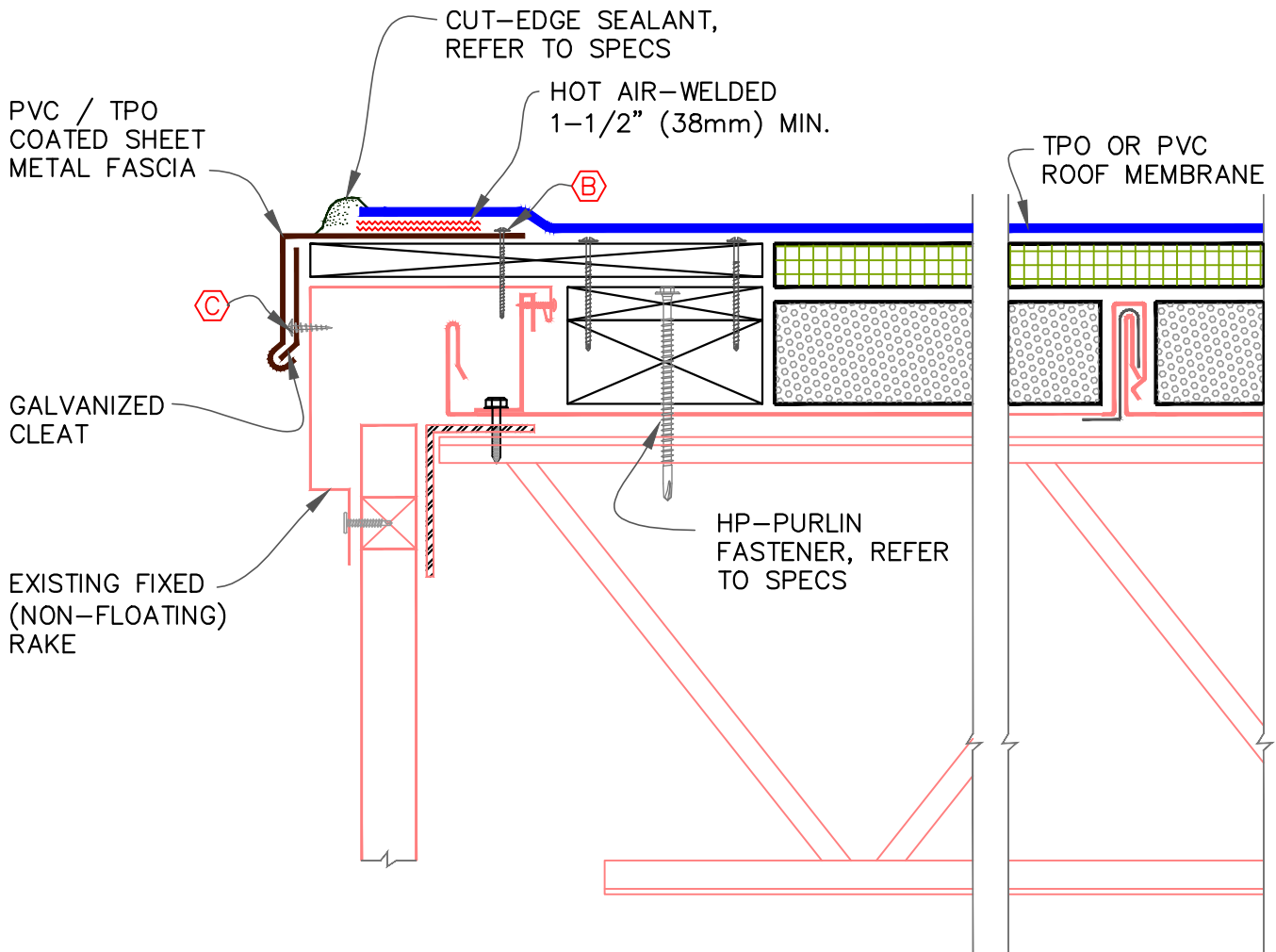
EXISTING FIXED RAKE EDGE
